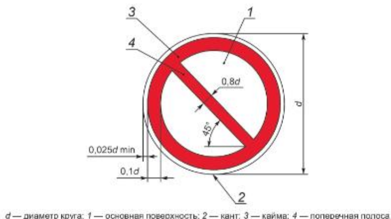
Рисунок 1 - Основа цветографического изображения и соотношение размеров
