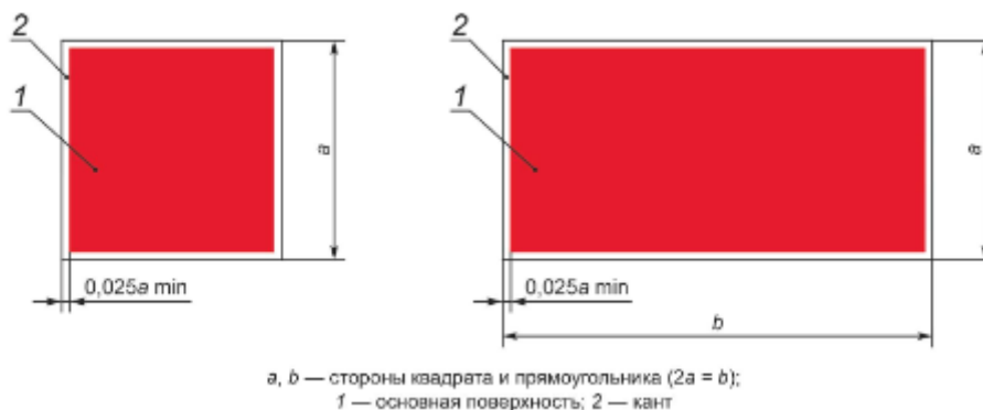
Рисунок 4 - Основа цветографического изображения и соотношение размеров знаков пожарной безопасности
