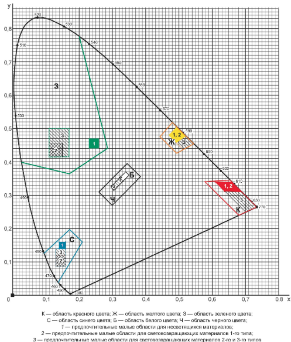
Рисунок А.1 - Допустимые области цветности x , y сигнальных и контрастных цветов на стандартном цветовом графике МКО 1931 г.
