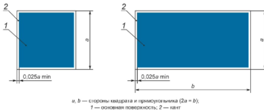
Рисунок 6 - Основа цветографического изображения и соотношение размеров указательных знаков безопасности
